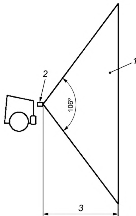
1 — зарегистрированный угол и сектор; 2 — камера; 3 — дальность в метрах
