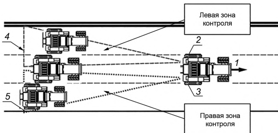
Рисунок 2 — Зоны контроля подсистемы обнаружения
