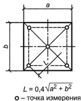
Рисунок 2 — Координаты точек измерения скорости воздушного потока
