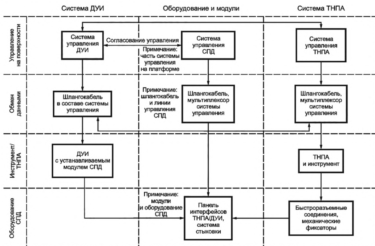
Рисунок 4 — Взаимосвязь между системами управления ДУИ, СПД и ТНПА, требуемые интерфейсы для совместного выполнения работ
