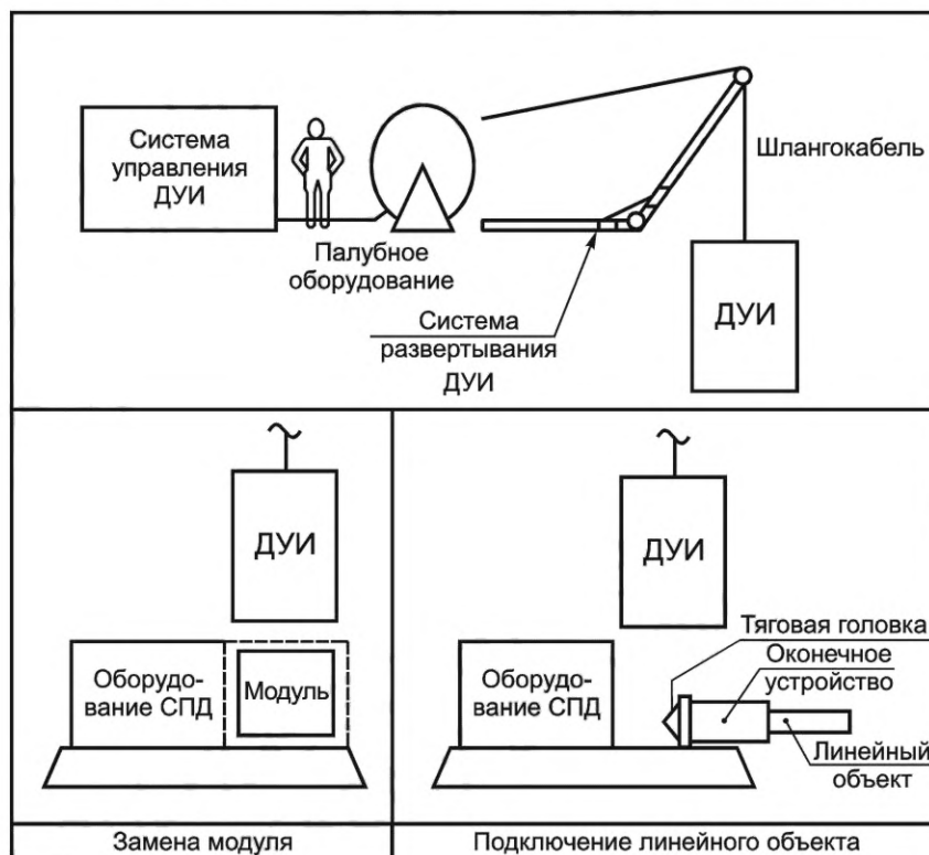
Рисунок 2 — Принципиальная схема выполнения работ на оборудовании СПД с применением ДУИ
