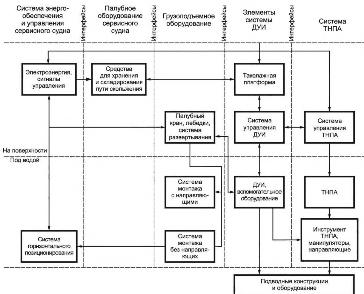
Рисунок 3 — Схема взаимодействия между сервисным судном, системой ДУИ и ТНПА
