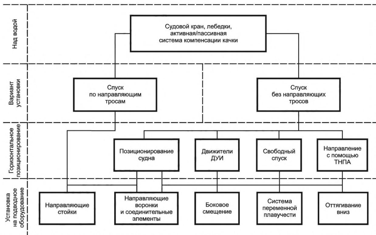
Рисунок 5 — Схемы развертывания системы ДУИ
