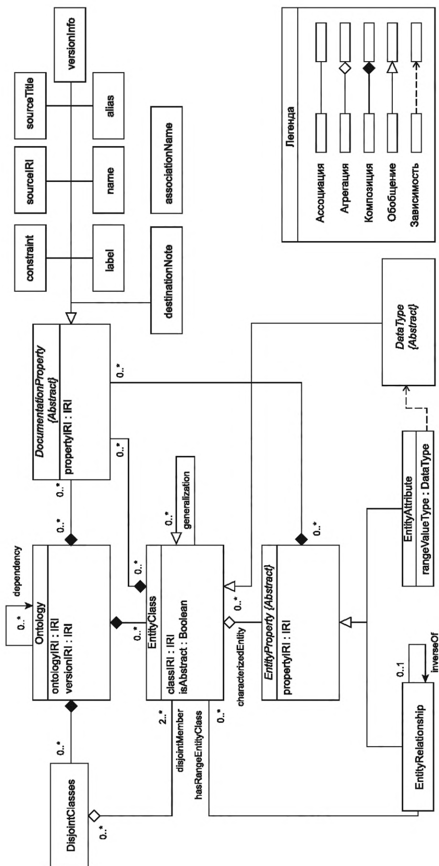
Рисунок 1 — UML-диаграмма информационной модели ОПО (расшифровка части обозначений приведена в таблицах 1—6)
