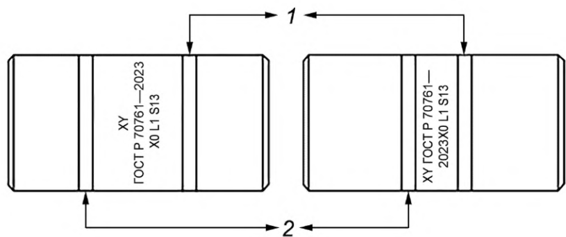
1 — полоса голубой краской на муфте с уплотнительными кольцами; 2 — полоса(ы) для групп прочности или другие полосы Рисунок D.29 — Пример расположения полос в цветовой маркировке муфты с уплотнительными кольцами
