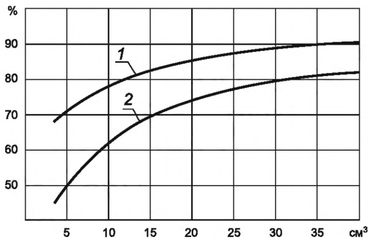
Рисунок 1 — Зависимость минимально допустимого значения коэффициента подачи и общего КПД пластинчатых насосов от рабочего объема в диапазоне от 3,2 до 40,0 см³
