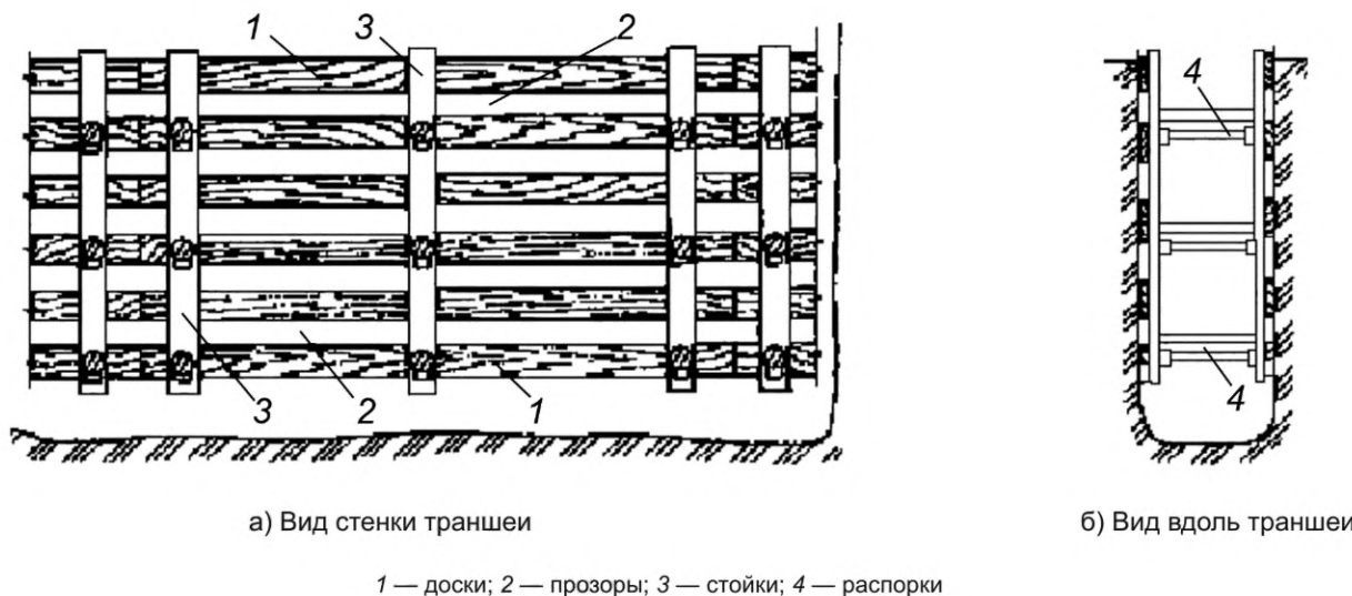
Рисунок Г.1 — Горизонтальное крепление стенок прямоугольной траншеи для укладки ПВ и ПТНК из ВЧШГ вразбежку
