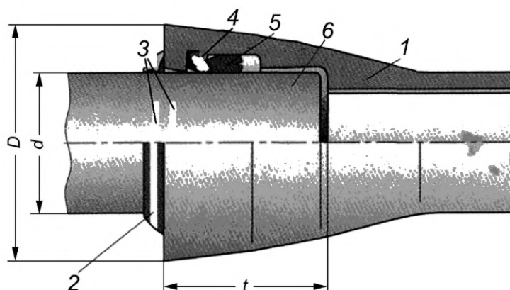
D, d — наружные диаметры раструба и трубы; t — глубина раструба; 1 — раструб; 2 — защитный замок; 3 — метки; 4 — пластина; 5 — РУМ с закладными металлическими пластинами; 6 — гладкий конец с фаской
