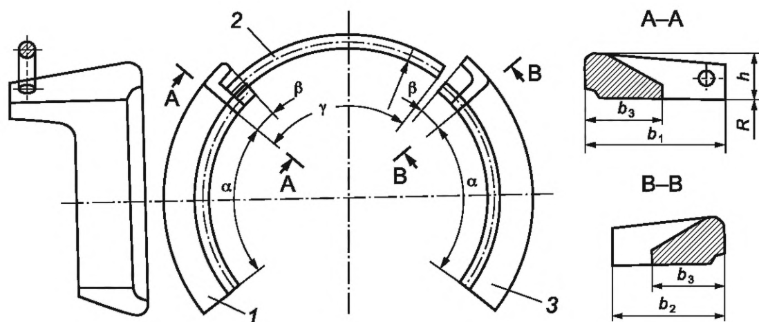
1, 3 — левый и правый стопоры; 2 — проволока; R — внутренний радиус стопора; b_1, b_2, b_3, h, \alpha, \beta, \gamma — конструктивные размеры стопора
