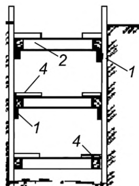
б) Вид вдоль траншеи
