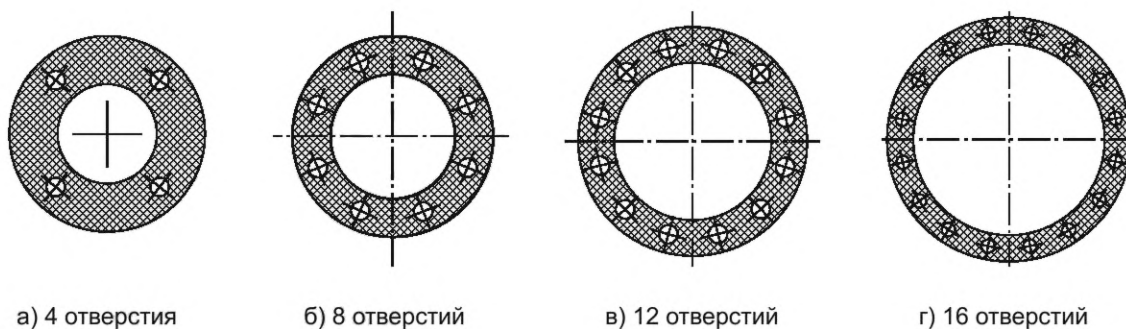
Рисунок 7.10 — Расположение отверстий в плоских прокладках для фланцевых соединений ТИ из ВЧШГ
