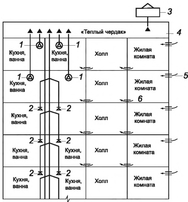
1 — индивидуальный вытяжной вентилятор; 2 — вытяжная решетка; 3 — вытяжная шахта с дефлектором; 4 — «теплый чердак»; 5 — приточный регулируемый клапан; 6 — переток
