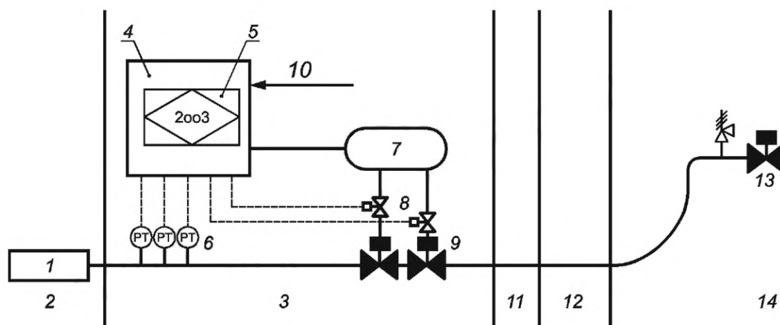
1 — пластовый флюид; 2 — залежь углеводородов как источник повышенного давления; 3 — ВИСЗД; 4 — ПМУ; 5 — ПЭС, работающее по логике 2003; 6 — датчики давления/температуры; 7 — гидравлический аккумулятор; 8 — клапаны на гидравлической линии; 9 — отсечные клапаны; 10 — шлангокабель системы управления; 11 — усиленный участок трубопровода; 12 — трубопровод; 13 — запорная арматура на платформе или берегу; 14 — технологическое оборудование, расположенное на платформе или берегу
