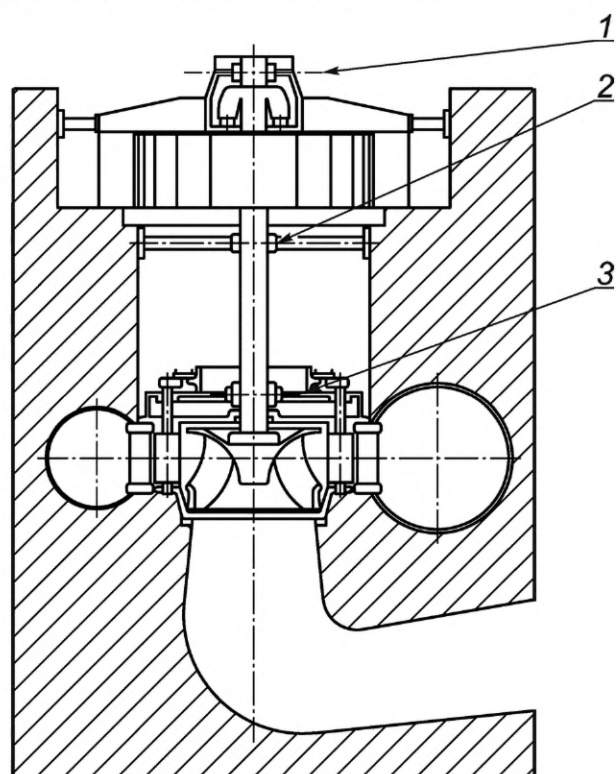
1 — направляющий подшипник, совмещенный с подпятником, в верхней крестовине генератора; 2 — направляющий подшипник в нижней крестовине генератора; 3 — направляющий подшипник турбины
