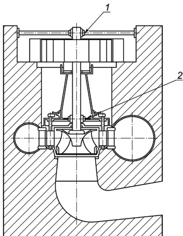
1 — направляющий подшипник генератора в верхней крестовине генератора; 2 — направляющий подшипник турбины
