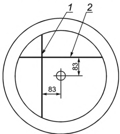
1 — первый шов для рулонов и плитки; 2 — второй шов для плитки
