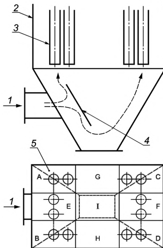
b — система рукавных фильтров с отражательной пластиной
