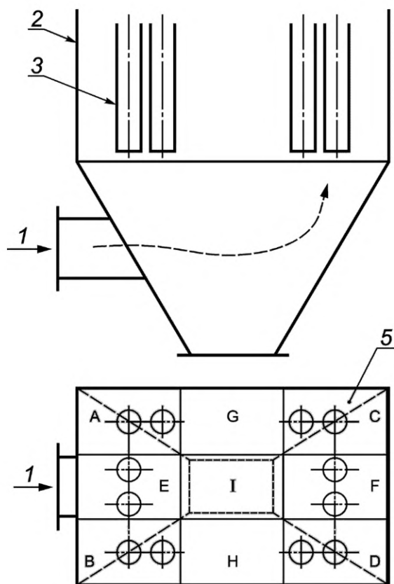
a — система рукавных фильтров без отражательной пластины
