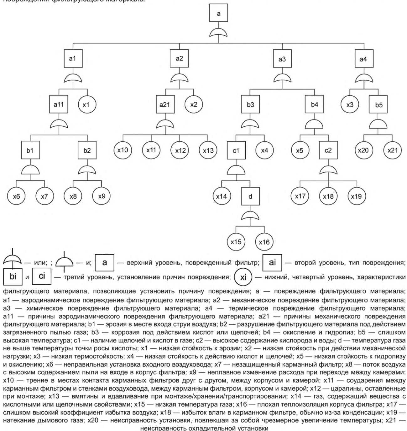
Рисунок А.1 — Анализ дерева неисправностей повреждения фильтра
