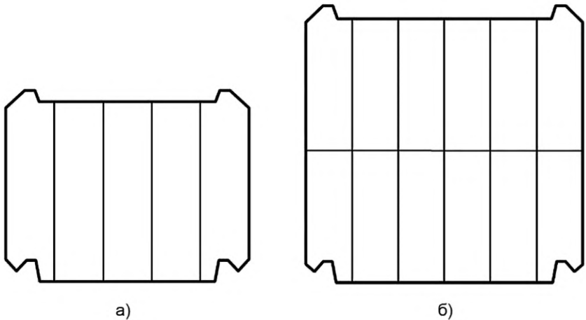
а) одноэтажный В1; б) склеенный из двух блоков — двухэтажный В2 Рисунок 2 — По количеству блоков склеивания
