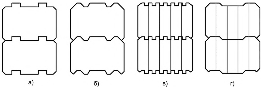
а) профиль с двумя шипами; б) профиль со скошенными шипами; в) «гребенка»; г) финский профиль Рисунок 1 —Типы клееного деревянного бруса по профилю
