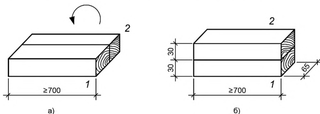
а) схема продольного распила; б) схема сборки; 1 и 2 — позиции ребер перед продольным распилом и после склеивания
