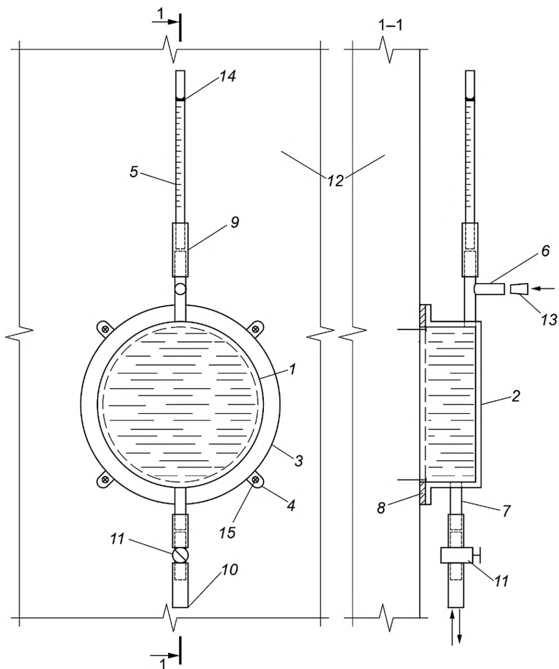
1 — камера металлическая; 2 — оргстекло; 3 — бортик; 4 — выпуски для крепления камеры к конструкции; 5 — мерная трубка; 6 — Т-образный штуцер для крепления мерной трубки; 7 — штуцер для подачи и слива воды; 8 — уплотняющее резиновое кольцо; 9 и 10 — силиконовые трубки; 11 — кран; 12 — конструкция; 13 — пробка; 14 — машинное масло; 15 — саморез
