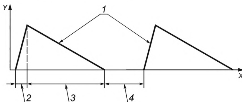
Рисунок 1 — Огибающая сигнала
