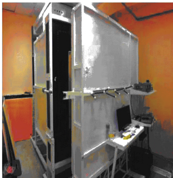
Рисунок 1 — Схема и фото установки для определения коэффициента теплопередачи образцов оконных и дверных блоков
