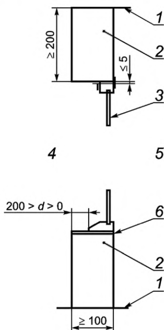
1 — граница области измерения; 2 — перегородка, \lambda \leq 0,04 Вт/(м · К); 3 — оконный блок; 4 — холодная сторона; 5 — теплая сторона; 6 — лицевая стенка профиля
