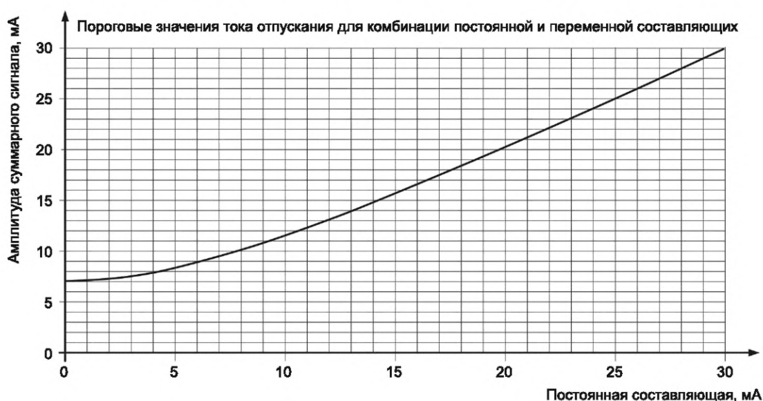
Рисунок 9 — 99,5 перцентилей порогового значения тока отпуска для комбинации тока частотой 50/60 Гц и постоянного тока
