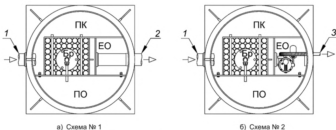
Рисунок 8 — Компоновочные схемы установок (тип Б)
