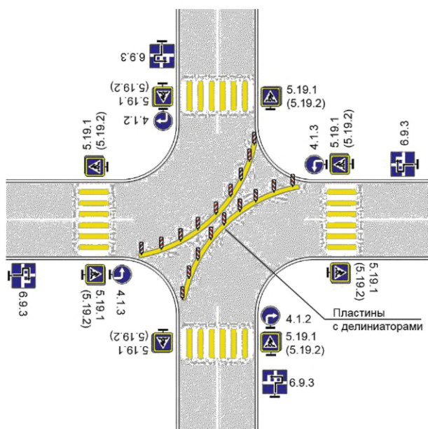
б) Установка делинаторов и дорожных пластин
