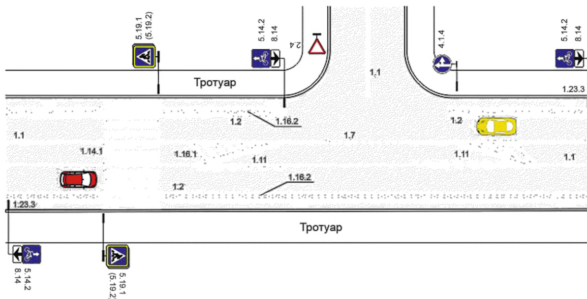
Рисунок Б.20 — Уменьшение ширины проезжей части с устройством велополос и выделением полосы для поворота налево
