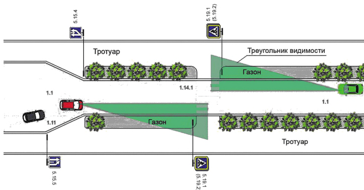
Рисунок Б.24 — Уменьшение числа полос с уширением тротуаров и устройством газонов и зеленых насаждений
