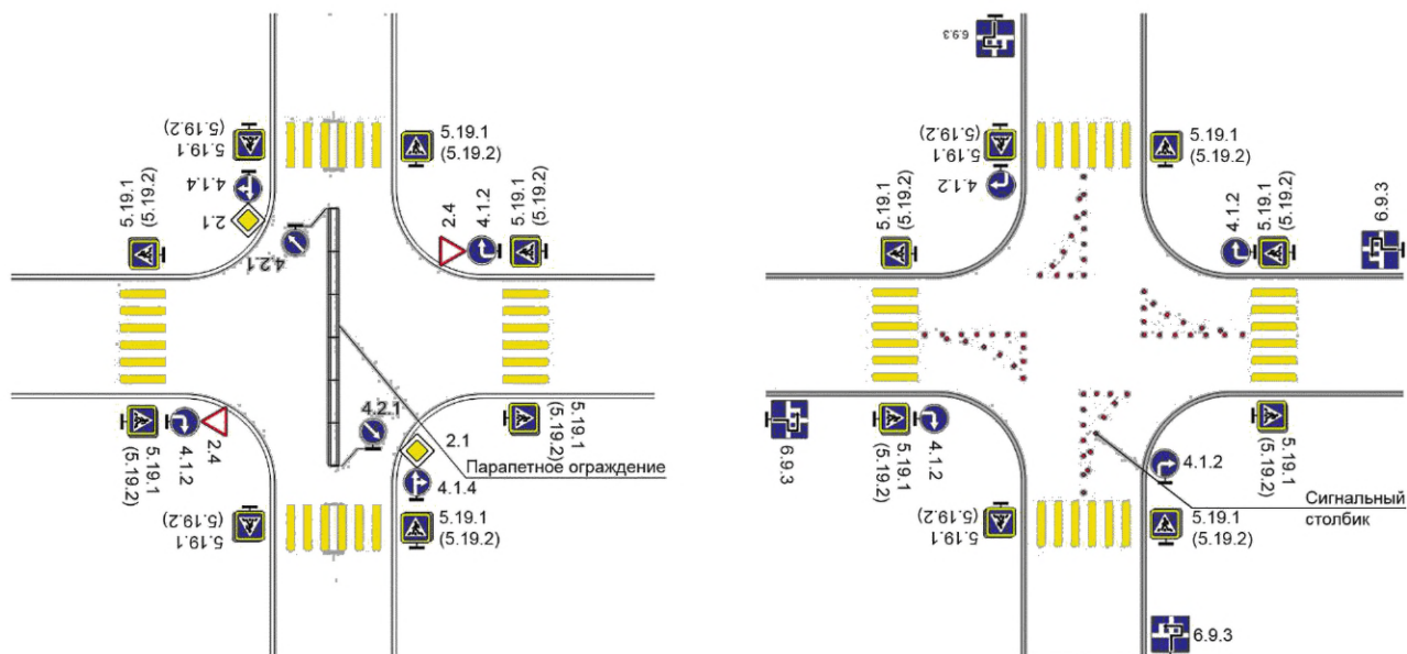
г) Перекрытие сквозного движения при помощи парапетного ограждения
