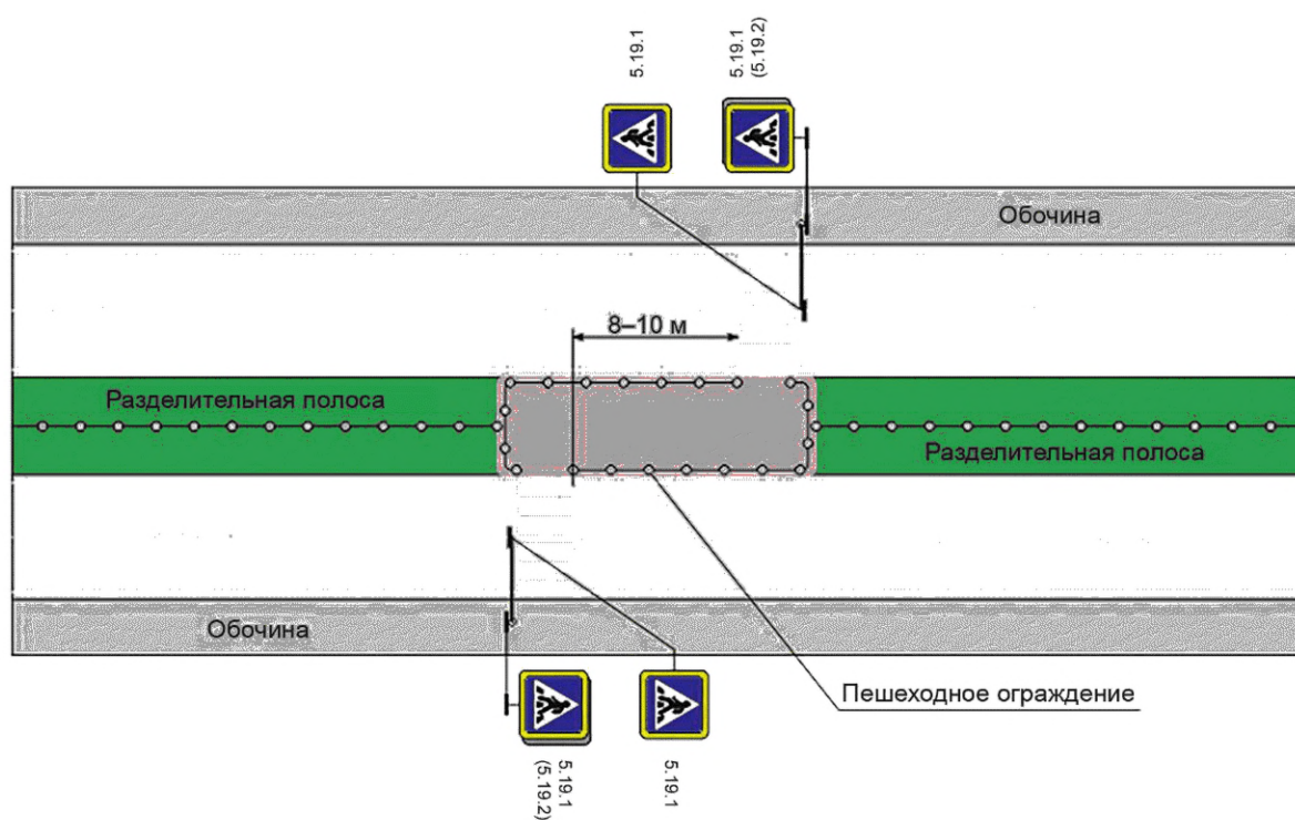
Рисунок Б.10 — Z-образный пешеходный переход с устройством ограничивающего пешеходного ограждения
