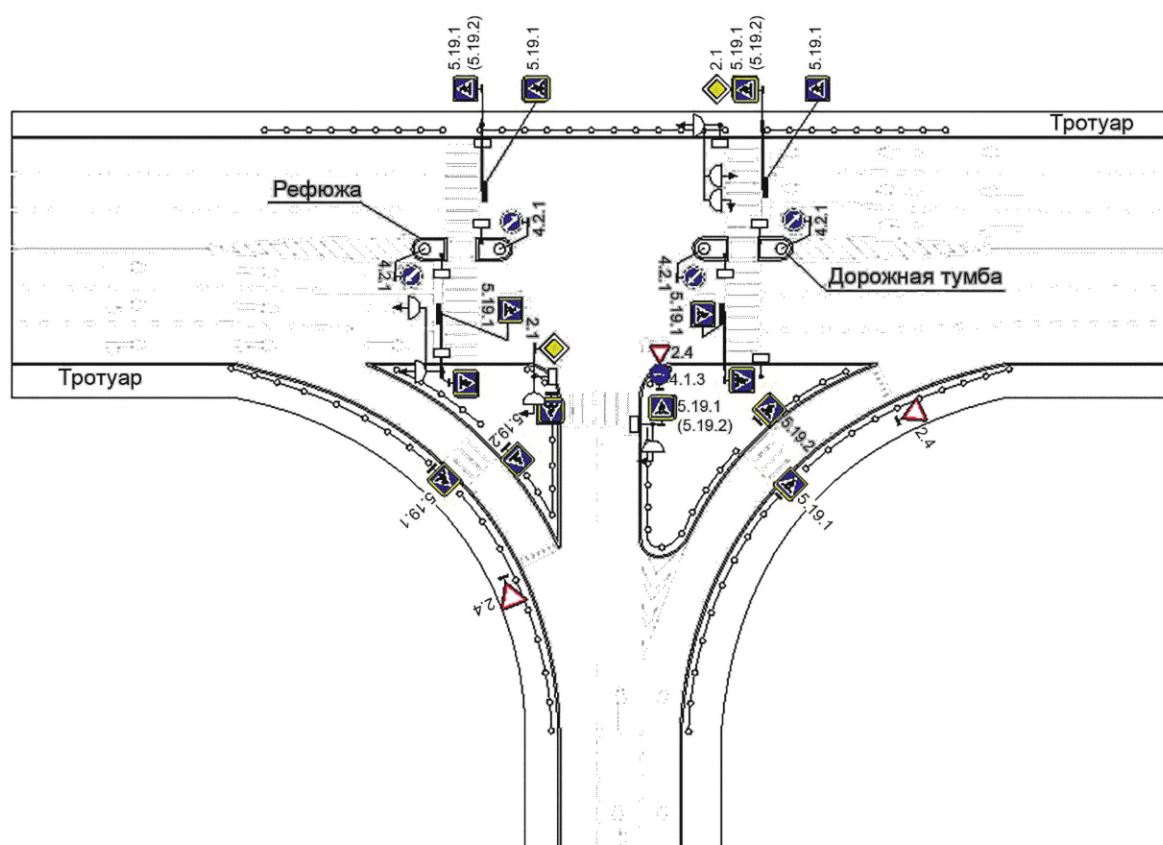
Рисунок Б.25 — Пример использования направляющих островков для перехода пешеходов на Т-образном пересечении
