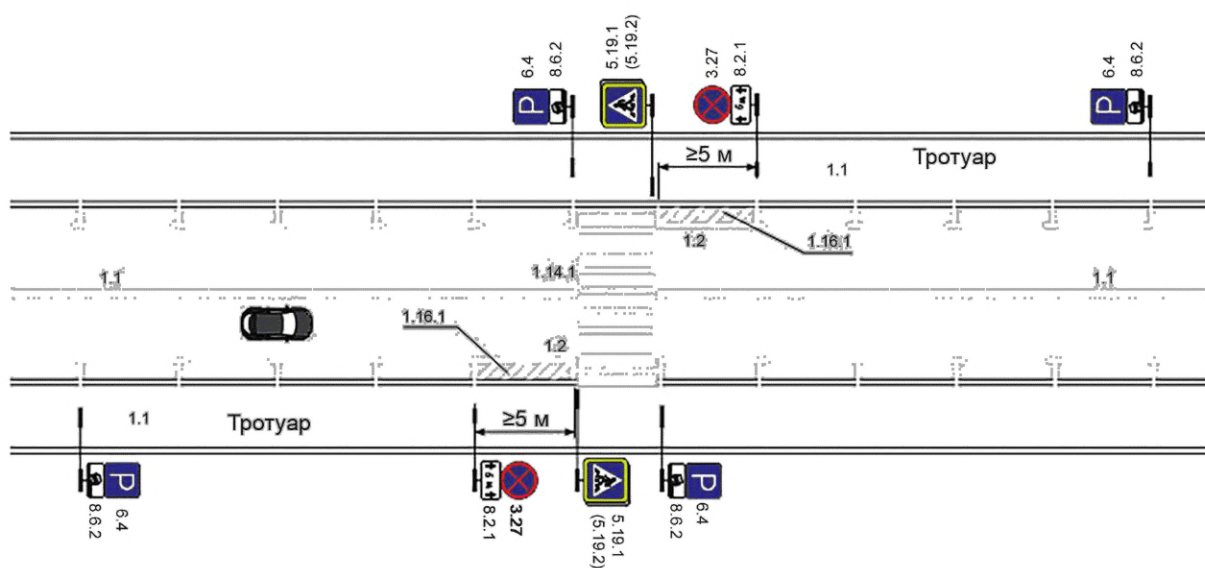
Рисунок Б.23 — Устройство парковочных мест с частичным использованием тротуара
