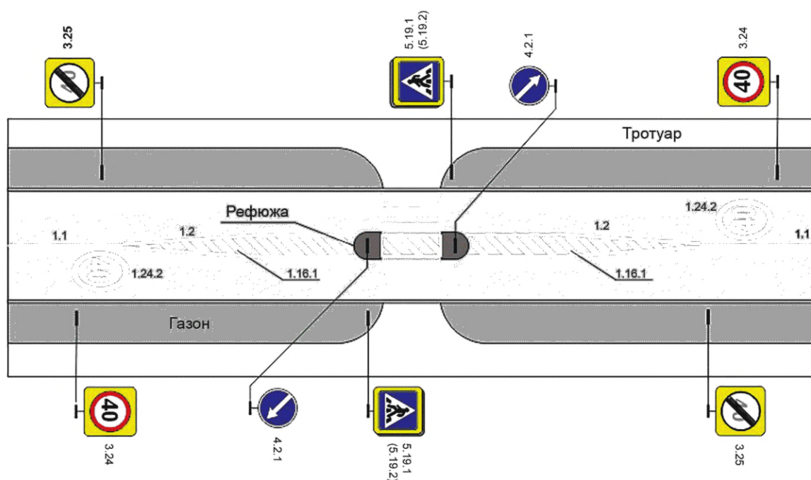
а) Без дорожной тумбы
