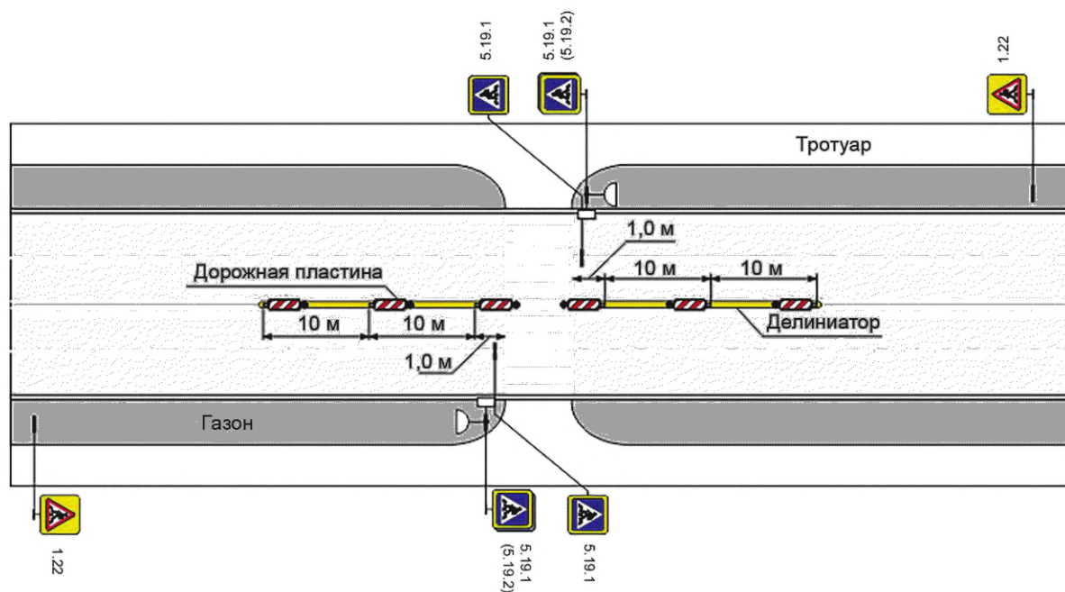
Рисунок Б.12 — Пример устройства защитных элементов на улицах с двумя полосами движения при помощи делиниаторов с дорожными пластинами
