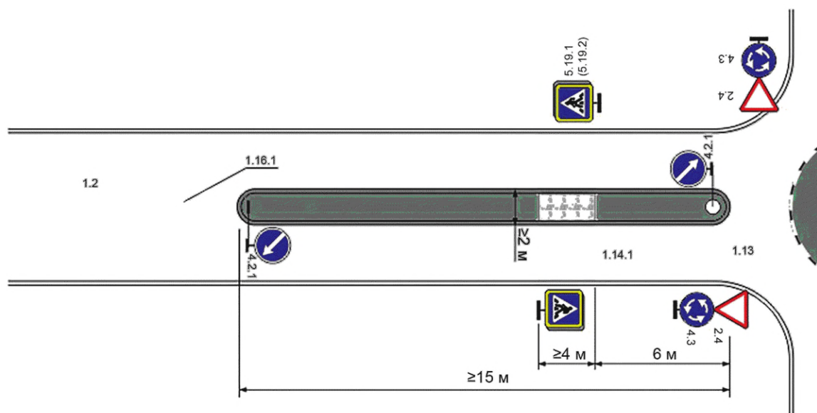
Рисунок Б.19 — Расположение и минимальные размеры островка безопасности для ожидания пешеходов
