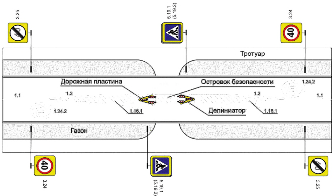
Рисунок Б.14 — Пример обустройства пешеходного перехода сигнальными пластинами на улицах с четырьмя полосами движения
