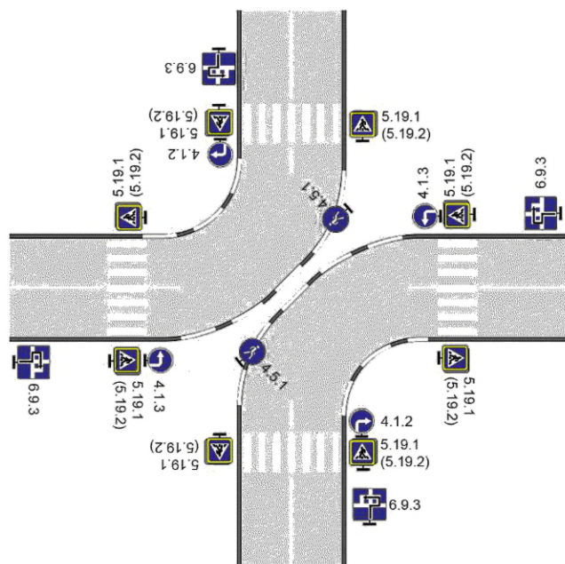
а) Устройство островка, приподнятого над проезжей частью, с движением пешеходов
