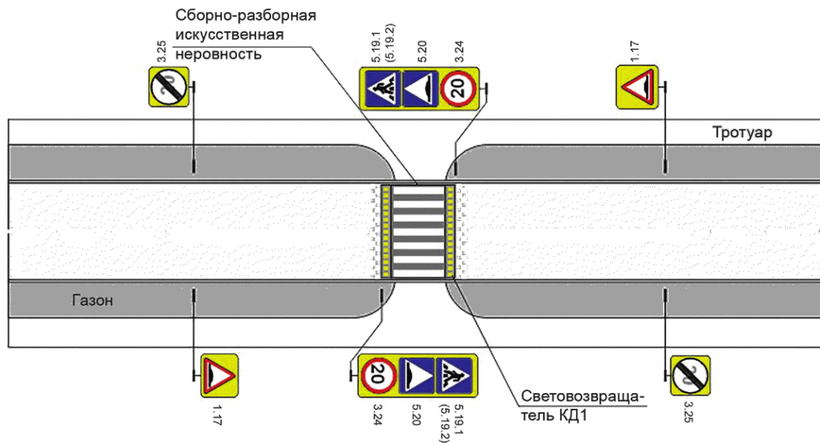
Рисунок Б.5 — Пример обустройства пешеходного перехода, совмещенного с искусственной неровностью
