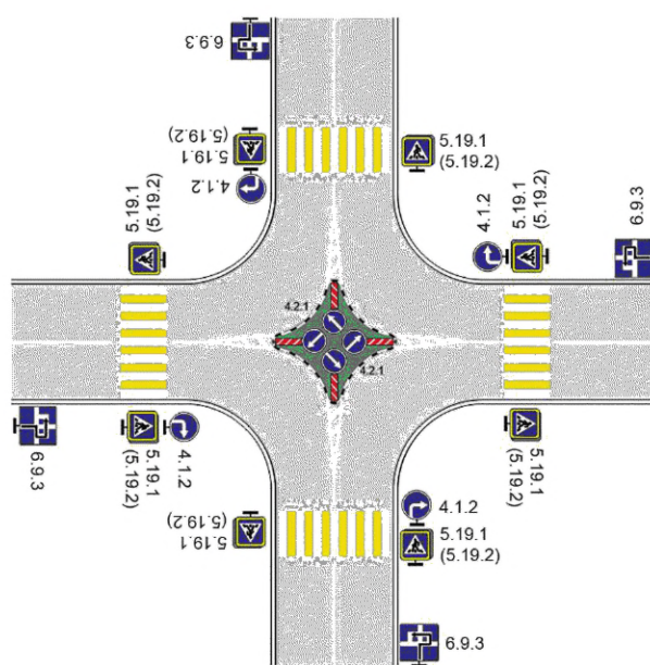
в) Устройство крестообразного направляющего островка, приподнятого над проезжей частью
