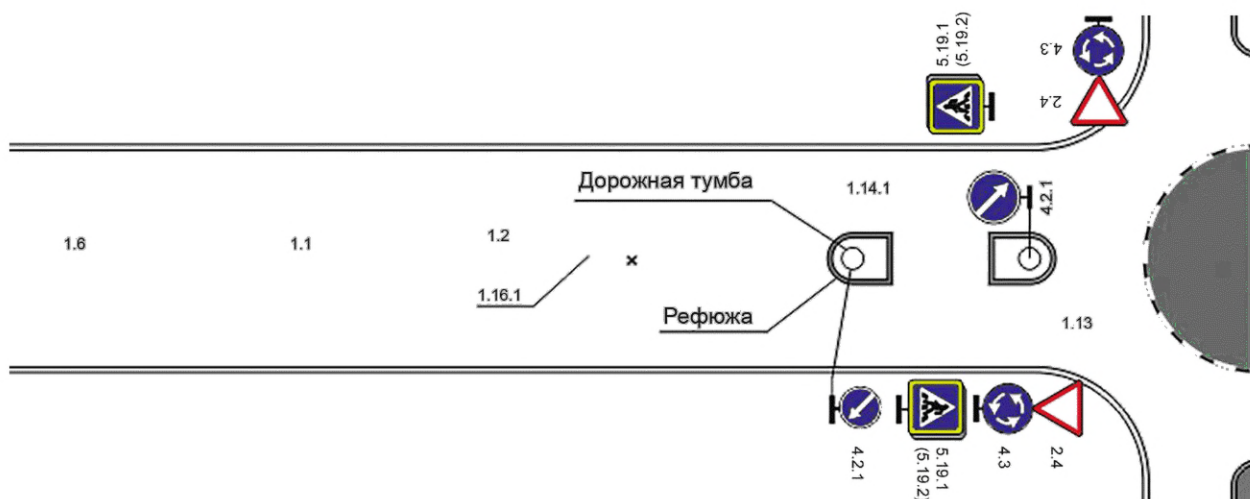
Рисунок Б.16 — Пример обустройства кольцевого пересечения пешеходными переходами и техническими средствами организации дорожного движения
