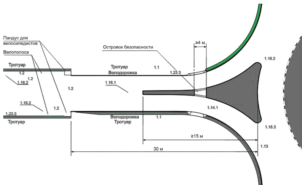
Рисунок Б.27 — Элементы кольцевого пересечения, обеспечивающие движение пешеходов и велосипедистов
