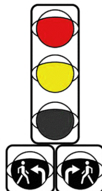
Рисунок Б.4 — Информационная световая секция, примеры размещения со светофором
