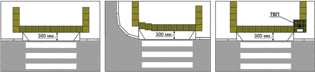
Рисунок Б.15 — Примеры обустройства пешеходных переходов наружными тактильными указателями
