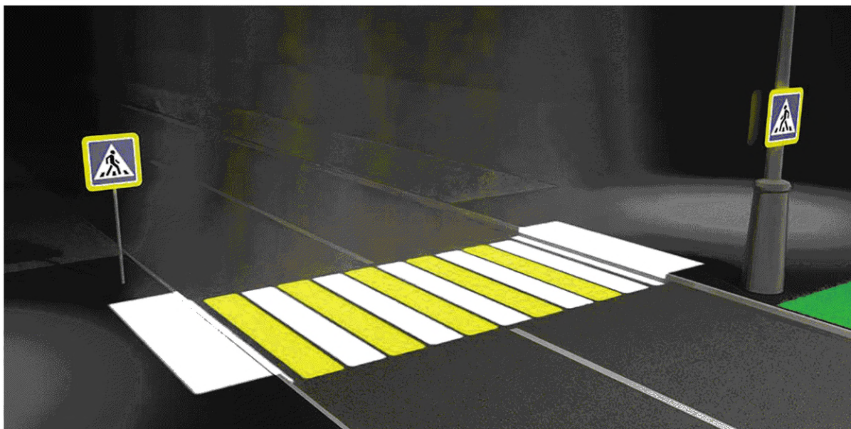
Рисунок Б.9 — Пример применения световой проекции разметки нерегулируемого пешеходного перехода и дополнительного освещения подходов к переходу
