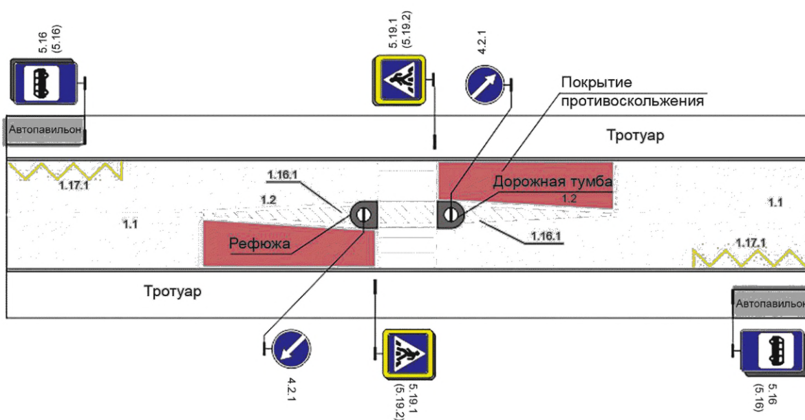
б) С дорожной тумбой в зоне остановочного пункта маршрутных транспортных средств
