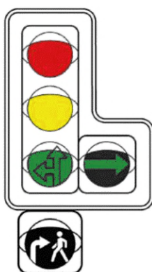
Рисунок Б.4 — Информационная световая секция, примеры размещения со светофором
