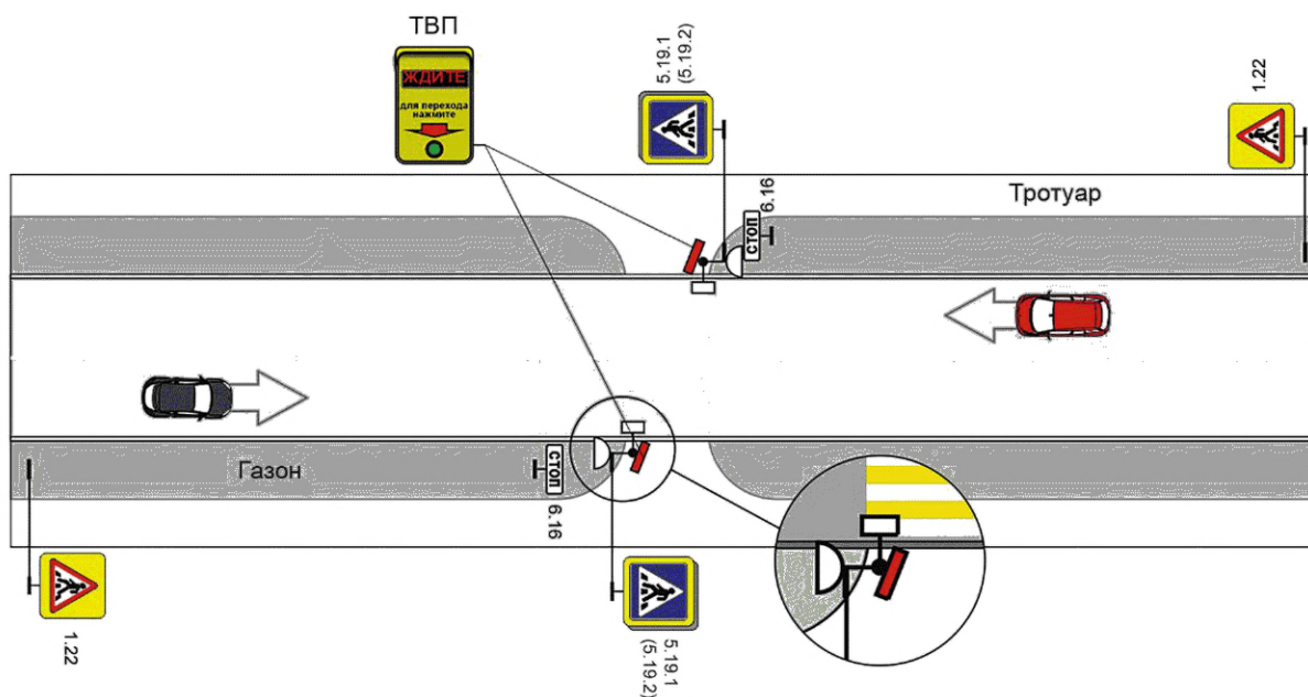
Рисунок Б.1 — Расположение ТВП (кнопки вызова) в направлении встречного движения (виден приближающийся транспорт)
