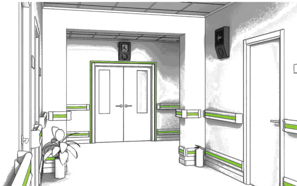
Рисунок А.3 — Пример размещения на стене и над дверью светозвуковых маяков для указания эвакуационного выхода и направления движения к нему, доступному для МГН, в том числе на креслах-колясках
