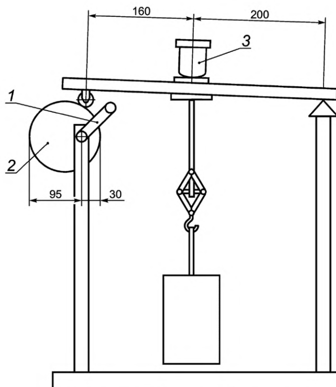
1 — ручка; 2 — эксцентрик; 3 — испытуемый образец
