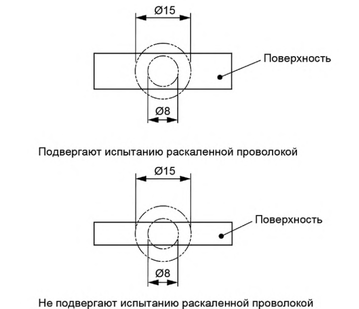
Рисунок 4 — Метод определения поверхности «мелких частей»
