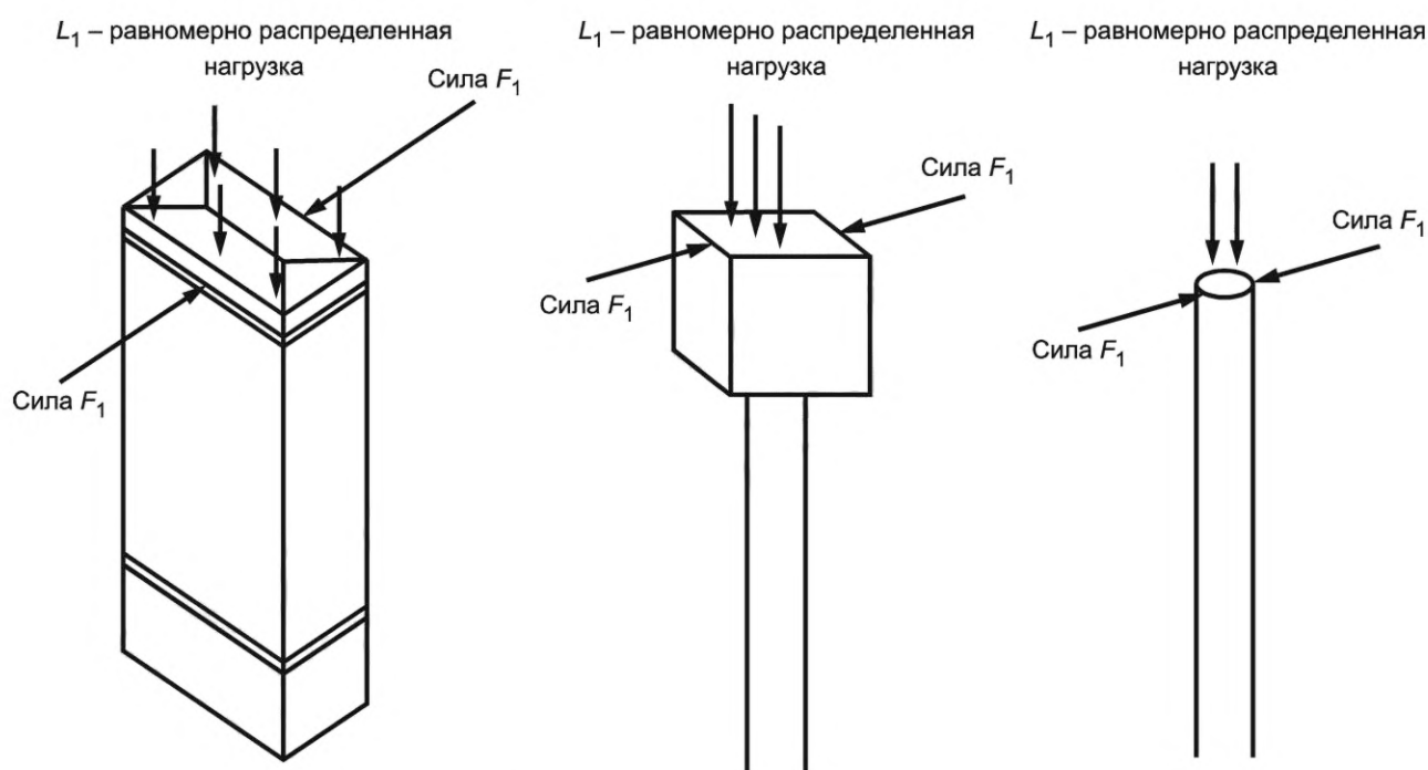
Рисунок 701 — Схема испытания стойкости к статической нагрузке
