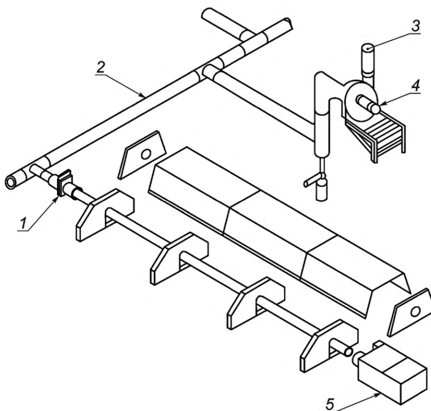
Рисунок В.8 — Системы типа D
