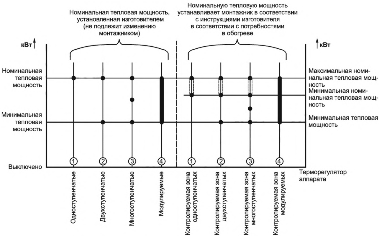
Рисунок G.1 — Обзор различных типов управления тепловой мощностью
