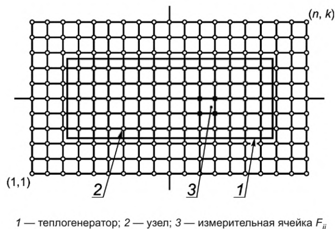
Рисунок 3 — Измерительная решетка
