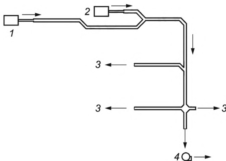
Рисунок В.7 — Общепринятая система D1
