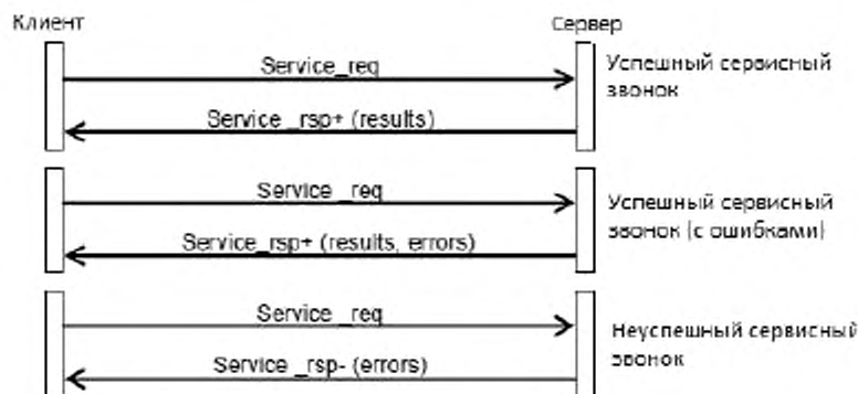
Рисунок 9 - Циклограмма
