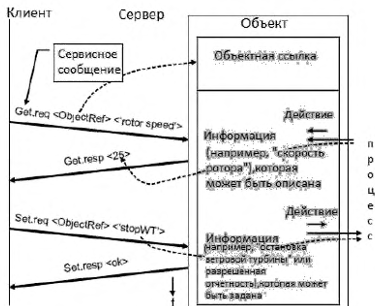
Рисунок 8 - IEC сервисная модель с примерами
