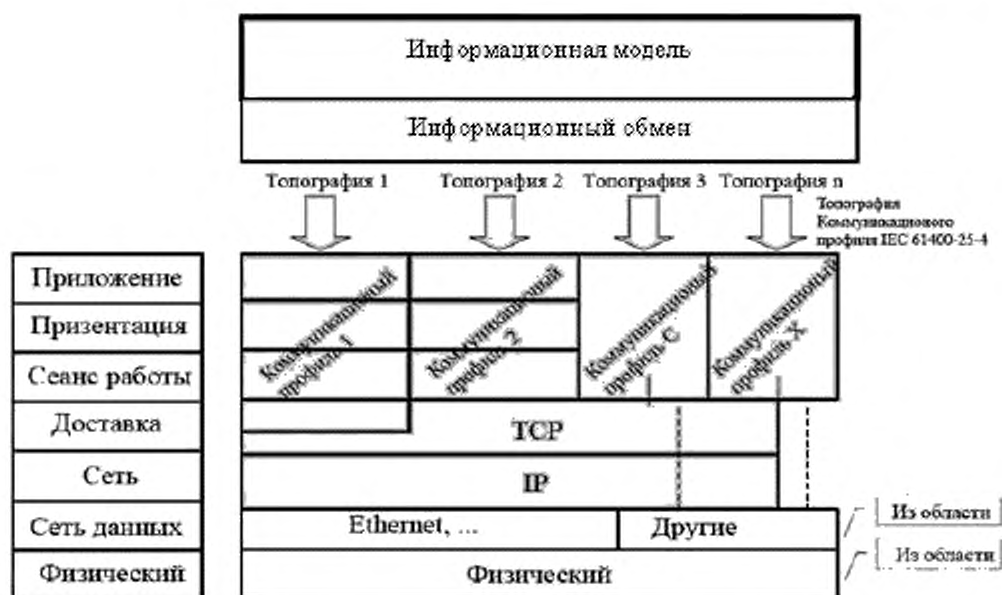
Рисунок 11 – Коммуникационные профили
