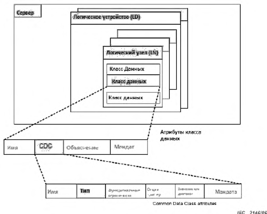
Рисунок 4 – Структура информационной модели ВЭС
