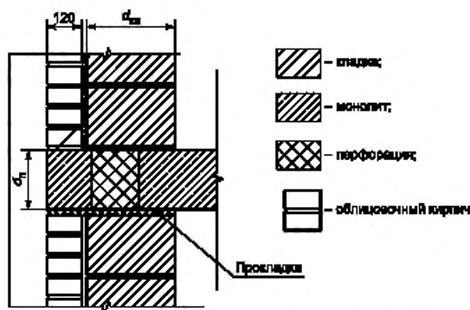
Рисунок А.1 — Схема узла сопряжения плиты перекрытия с наружной стеной
