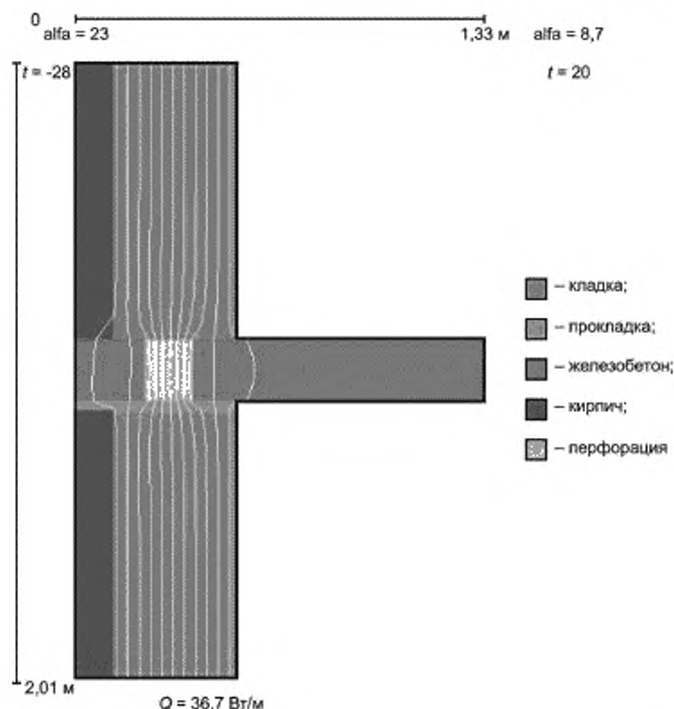
Рисунок А.2 — Температурное поле узла сопряжения плиты перекрытия с наружной стеной
