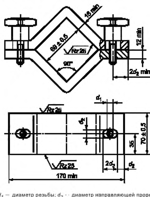
Рисунок 3 — Зажимная форма для установки кубической пробы
