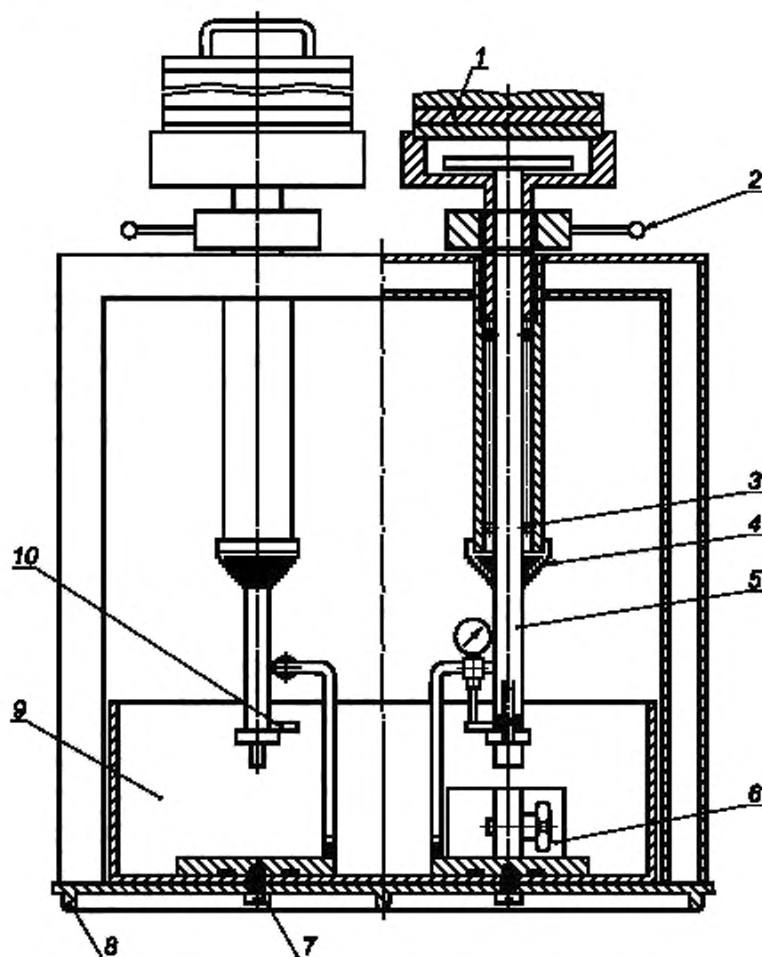
1 — гири-разновеска; 2 — подъемный механизм; 3 — шариковые втулки; 4 — защитный кожух; 5 — шток; 6 — зажимная форма; 7 — крепежный винт; 8 — ребро жесткости; 9 — водяная баня; 10 — контактная пластина индикатора часового типа
