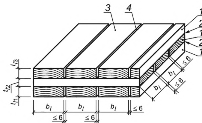
1 — слой древесины: 6 \leq (t_{11} \text{ и } t_{13}) \leq 45 , 6 \leq t_{12} \leq 60 , 60 \leq b_1 \leq 300 ; 2 — клеевые швы между слоями; 3 — заготовка; 4 — зазор между заготовками в слое; b_1 — ширина ламели; t_{11} , t_{12} , t_{13} — толщины слоев
