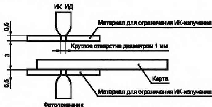
Рисунок 14 — Правильное расположение ИК ИД и фотоприемника
