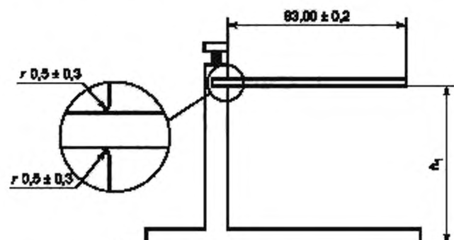
Рисунок 16 — Карта в зажимном устройстве до воздействия температуры
