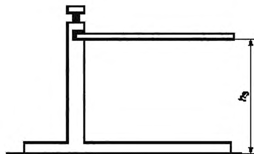
Рисунок 9 — Карта в зажимном устройстве после снятия нагрузки
