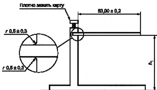
Рисунок 7 — Карта в зажимном устройстве до приложения нагрузки
