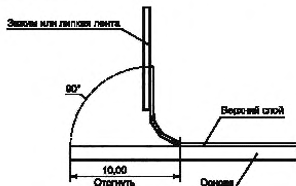
Рисунок 4 — Подготовка образца к испытанию
