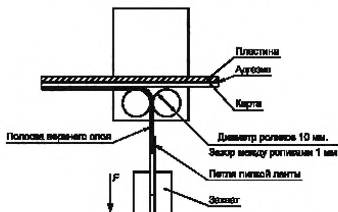
Рисунок 5 — Схема установки карты в разрывной машине
