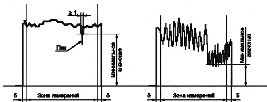
Рисунок 6 — Примеры диаграмм прочности сцепления
