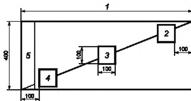
1 — ширина полотна материала; 2, 3, 4 — образцы, 5 — кромка
