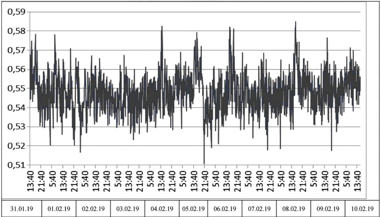
Рисунок 0.1.4 — График значений приведенного сопротивления теплопередаче оконного блока, м 2 · °C/Вт
