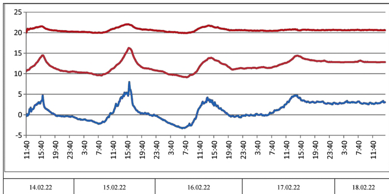
Рисунок А.9 — Графики значений температур внутреннего воздуха (верхняя линия), наружного воздуха (нижняя линия) и поверхности в точке a на стеклопакете, °C
