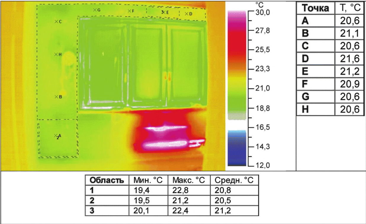
Рисунок 0.2.1 — Распределение температурных полей на испытываемой конструкции
