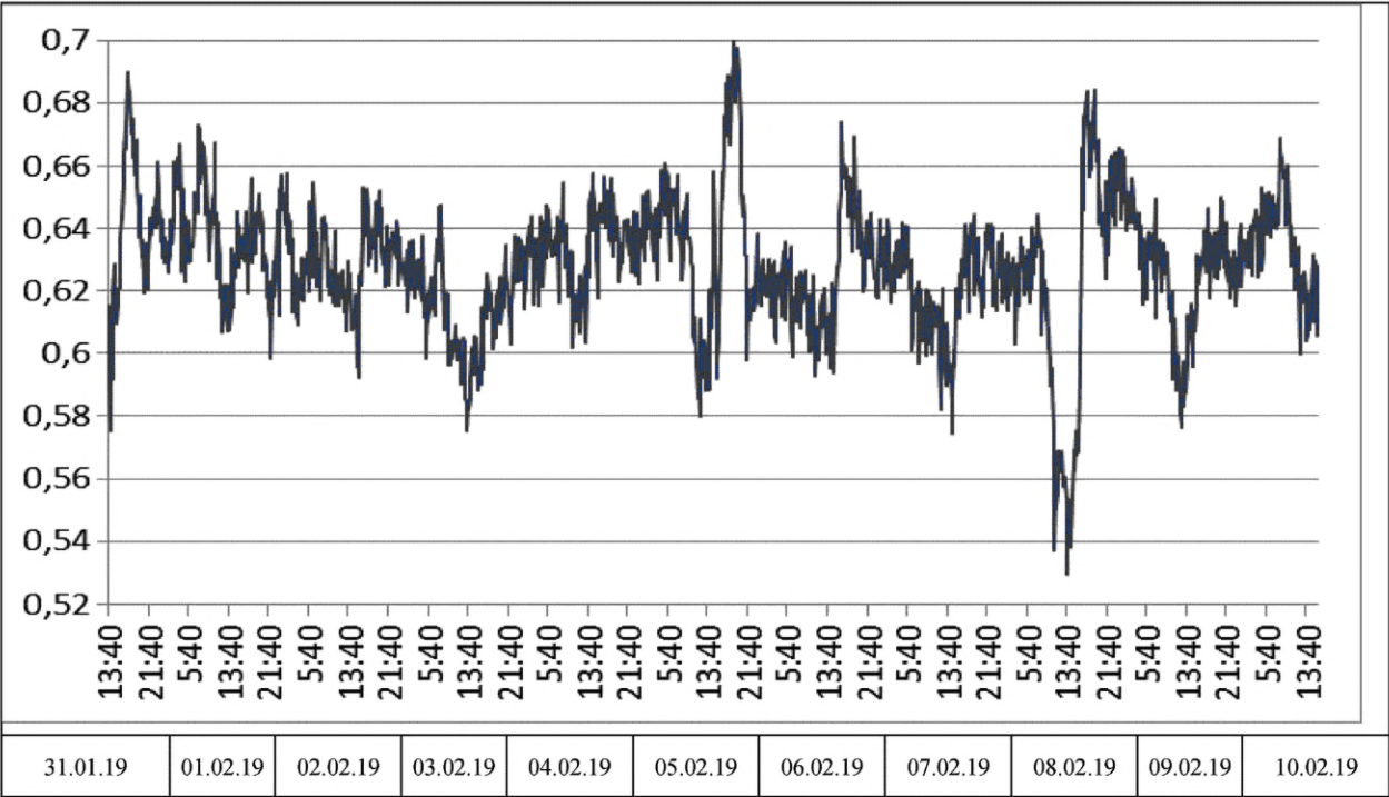
Рисунок 0.1.5 — График значений приведенного сопротивления теплопередаче профиля коробки, \text{м}^2 \cdot ^\circ\text{C}/\text{Вт}
