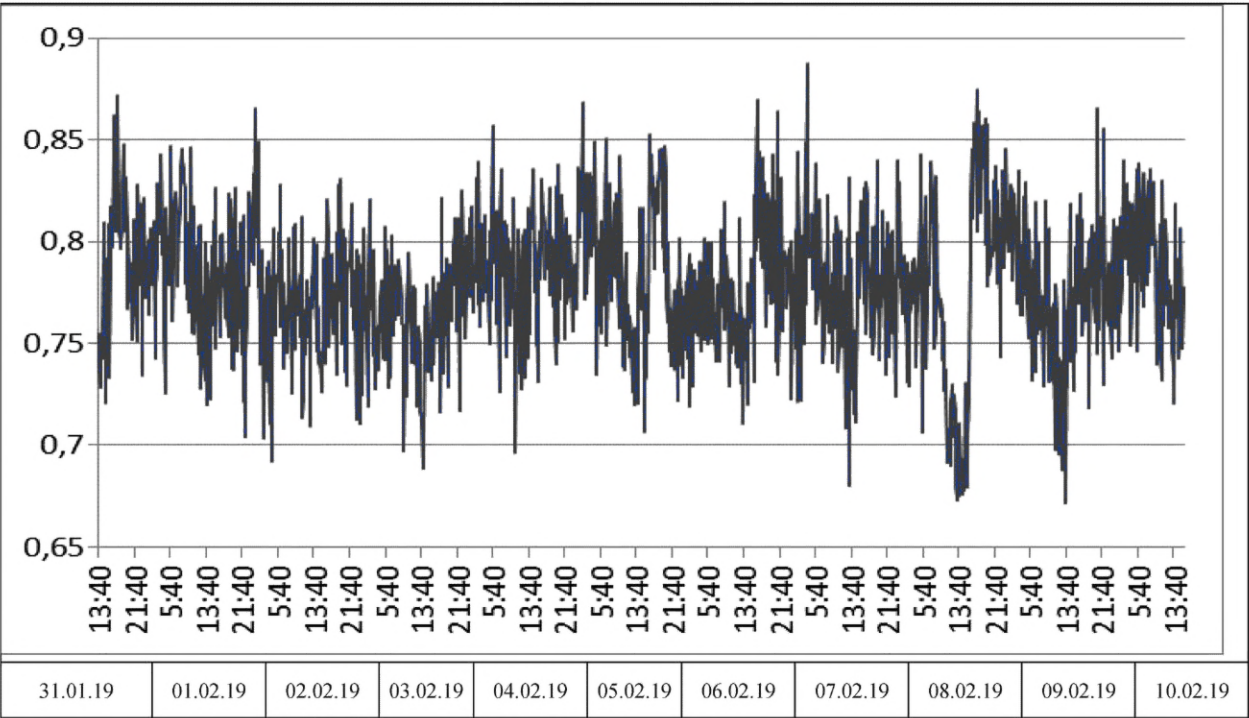
Рисунок 0.1.6 — График значений приведенного сопротивления теплопередаче профиля створок, \text{м}^2 \cdot ^\circ\text{C}/\text{Вт}
