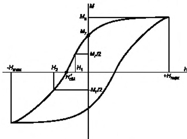
Рисунок 20 — Петля гистерезиса
