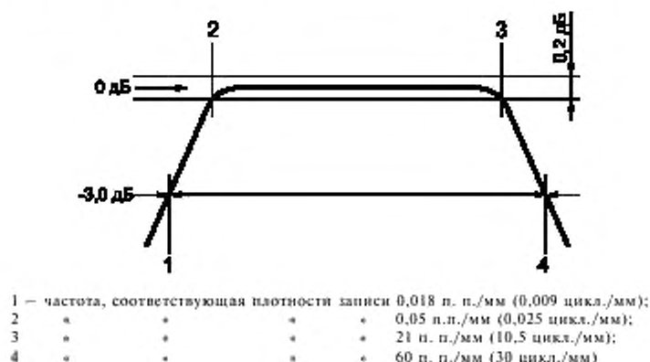
Рисунок 15 — Характеристика фильтра
