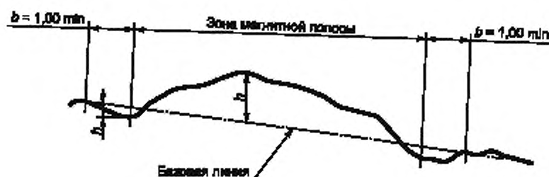
Рисунок 9 — Выпуклый профиль полосы
