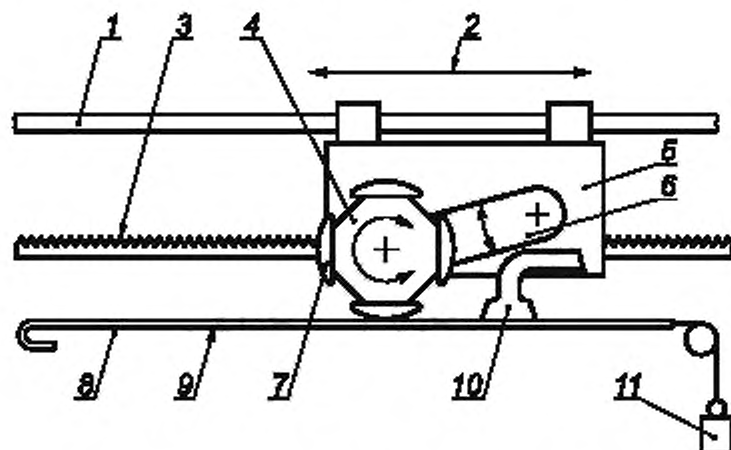
1 — направляющая планка; 2 — направление движения; 3 — зубчатая рейка; 4 — третрад; 5 — рама; 6 — кулиса; 7 — стопа; 8 — пылесос; 9 — проба; 10 — пылесос; 11 — предварительная нагрузка
