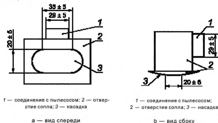
Рисунок 2 — Опора присоски
