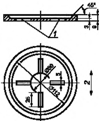
1 — радиус закругления всех граней диска > 0,5 мм; 2 — продольное направление образца
