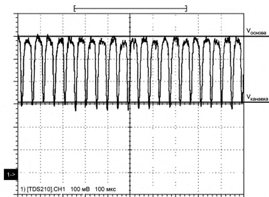
Рисунок 8 — Контраст направляющих дорожек
