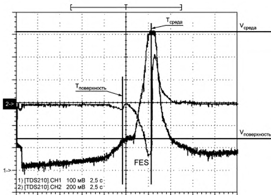
Рисунок 6 — Формы сигналов, получаемые при развертке по фокусу
