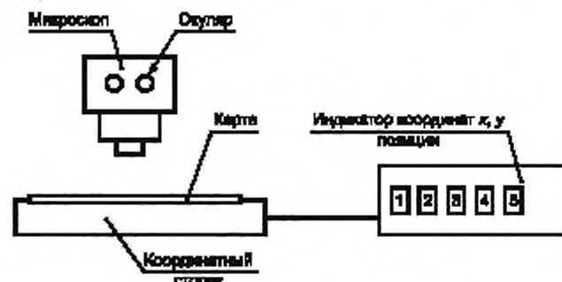
Рисунок 2 — Средства измерений наклона
