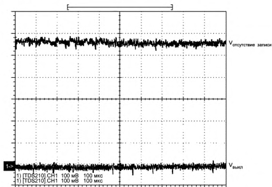
Рисунок 7 — RF уровни при отсутствии записи и выключенном лазере
