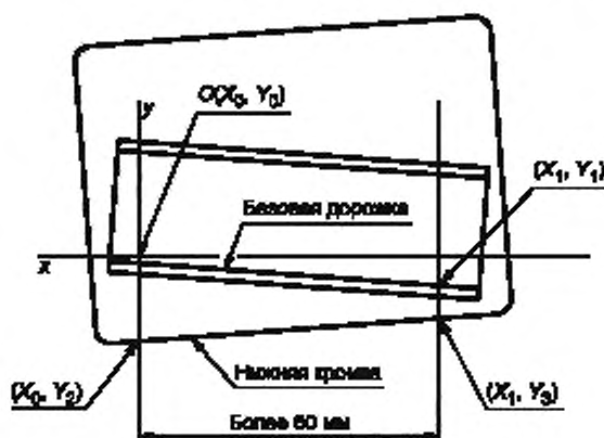
Рисунок 3 — Метод измерения наклона
