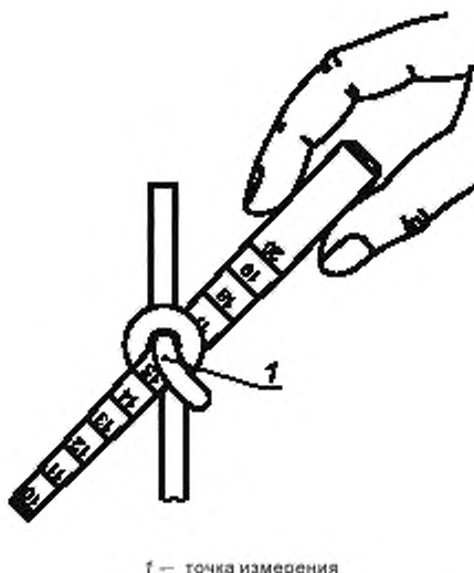
Рисунок 2 — Определение способности к вязке узлов K
