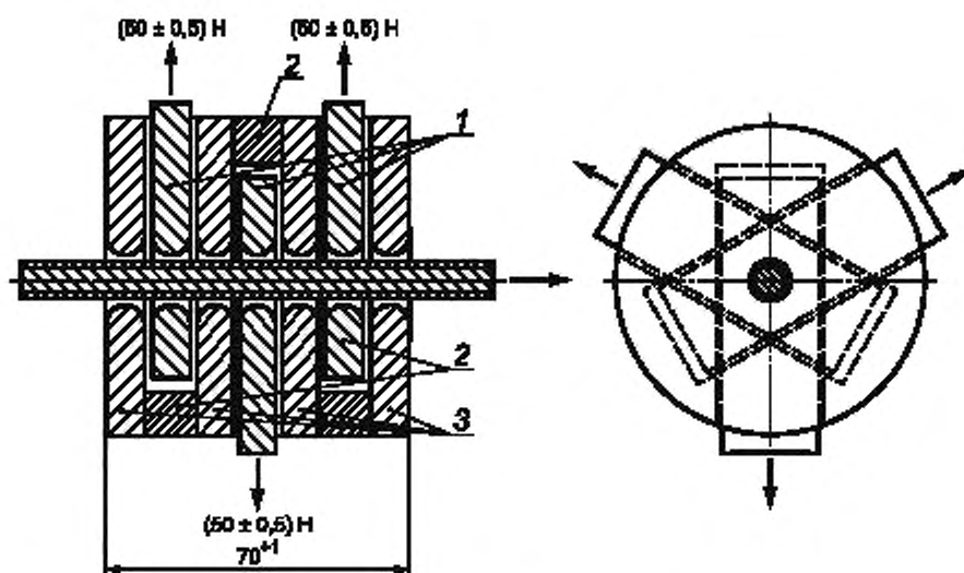
1 — движущие пластины, 2 — пространство; 3 — закрепленные пластины
