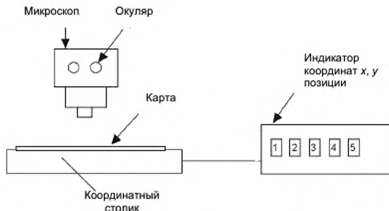
Рисунок 2 – Оборудование для измерения наклона
