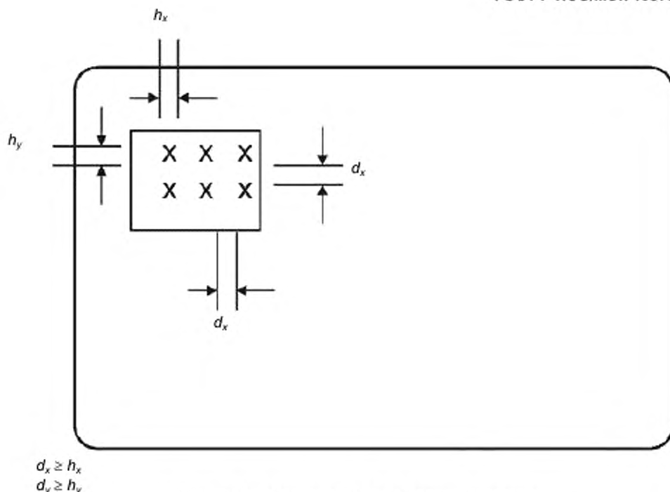
Рисунок 4 — Компоновка из нескольких голограмм
