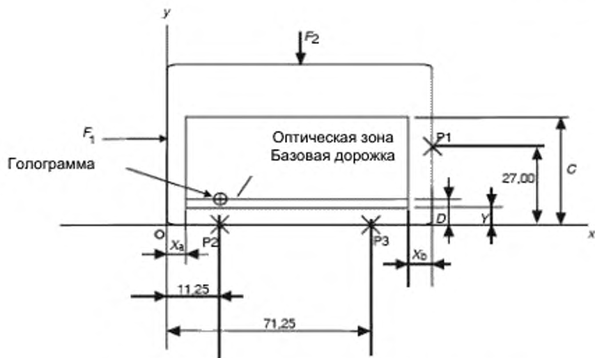
Рисунок 1 – Расположение оптической зоны и базовой дорожки
