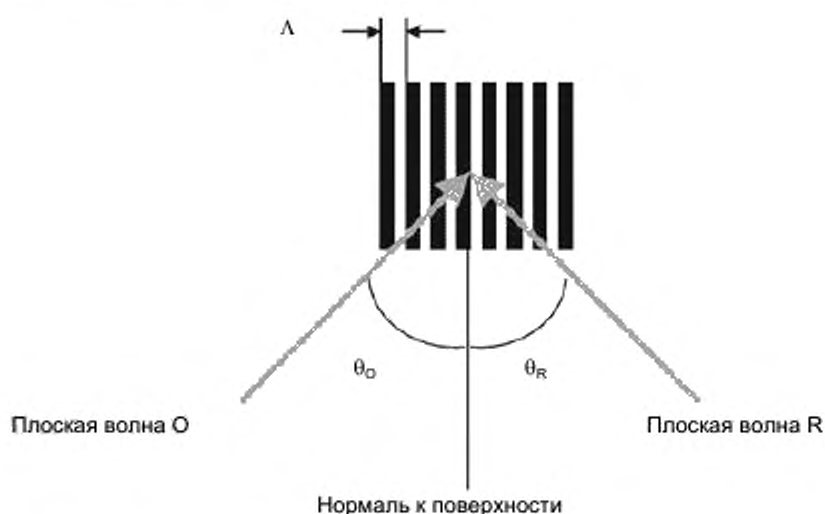
Рисунок 5 – Запись дифракционной решетки в запоминающем слое при помощи интерференции двух плоских волн
