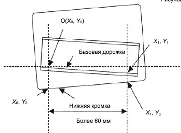
Рисунок 3 – Методика измерения наклона
