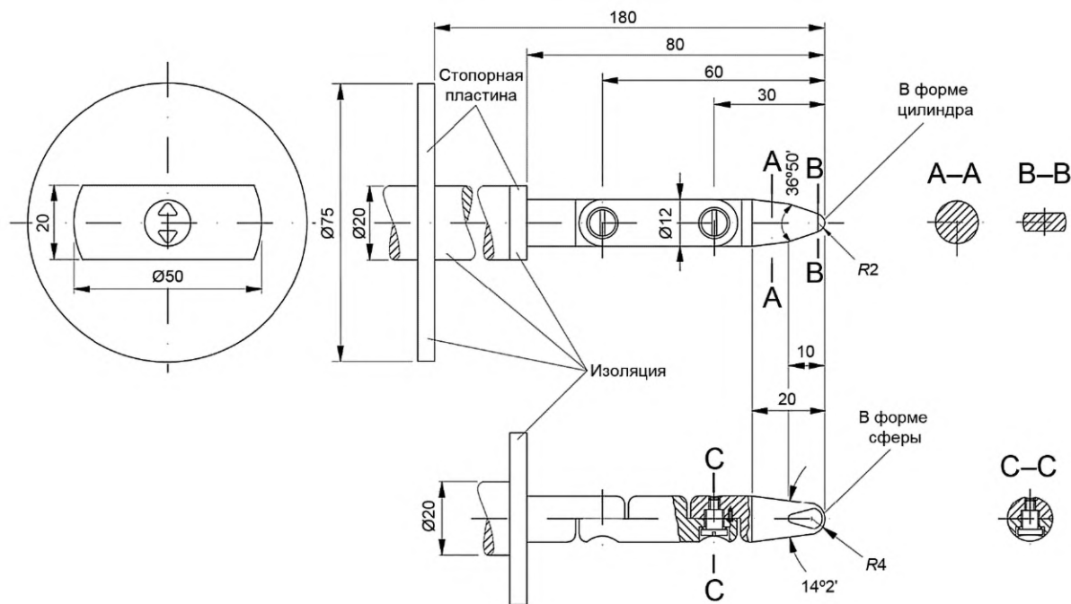
Рисунок 2 — Шарнирный зонд
