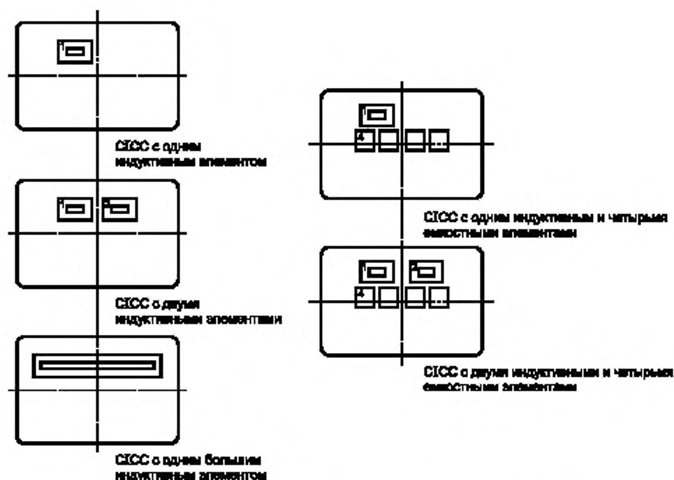
Рисунок Б.2 — Примеры вариантов компоновки элементов связи в СІС
