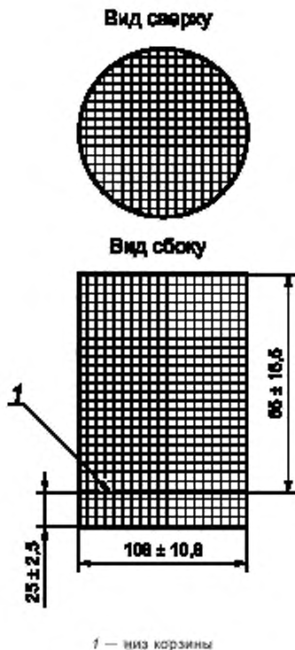
Рисунок 1 — Проволочная корзина
