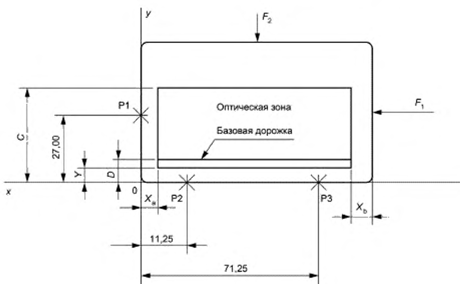
Рисунок 1 — Расположение оптической зоны и базовой дорожки
