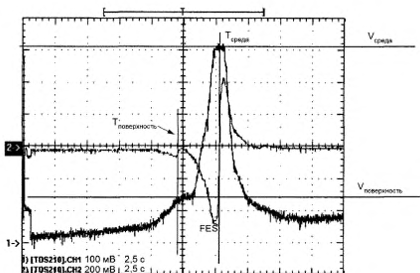
Рисунок 7 — Формы сигналов при развертке по фокусу
