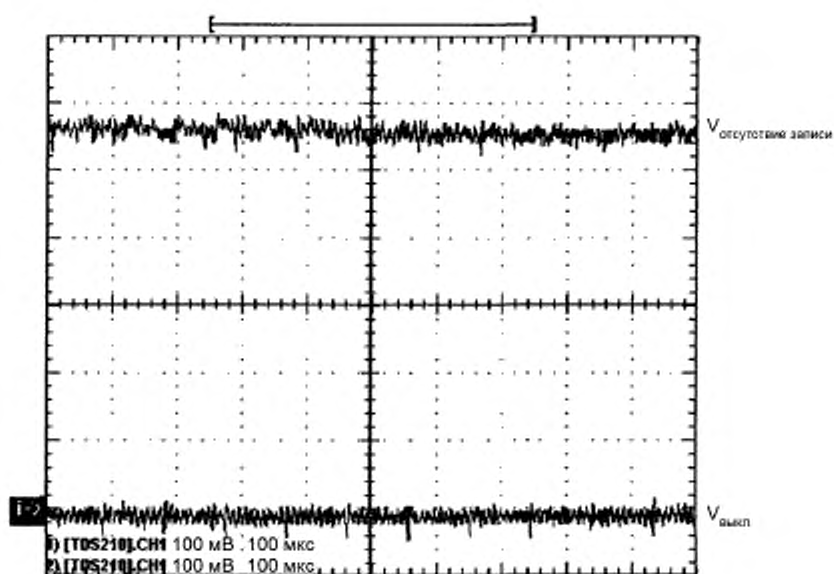
Рисунок 8 — RF уровни при отсутствии записи и выключенном лазере
