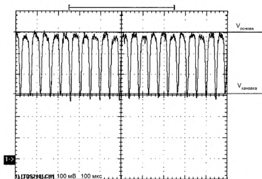
Рисунок 9 — Контраст направляющих дорожек
