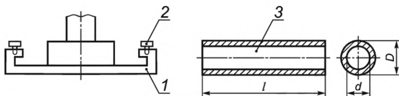
1 — основание для крепления шланга; 2 — винт для крепления; 3 — резиновый шланг с твердостью резины (80 \pm 2) IHRD, длиной l = (127 \pm 1) мм, наружным диаметром D = (30 \pm 1) мм и внутренним диаметром d = (19 \pm 0,5) мм
