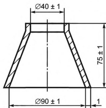
Рисунок 4 — Металлическая форма в виде конуса
