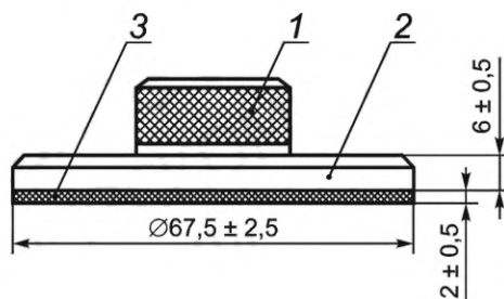
1 — рукоять; 2 — диск; 3 — резиновое покрытие
