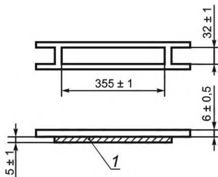
1 — уплотнитель
