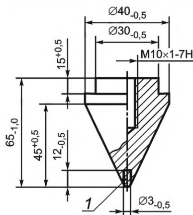
Рисунок 2 — Прибор для определения твердости дорожного покрытия
