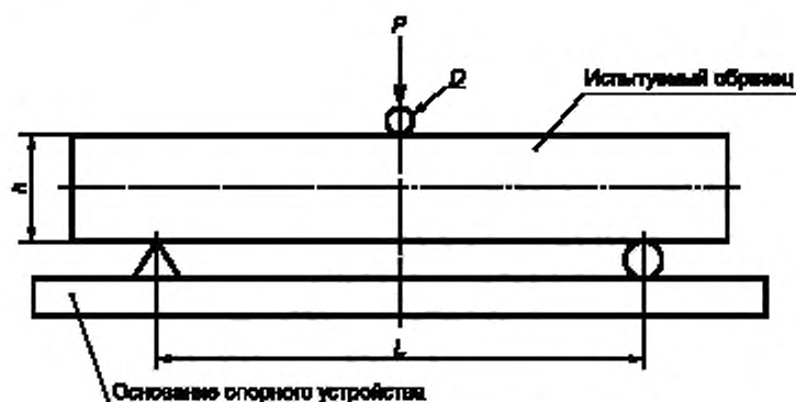
Рисунок 1 — Схема опорного устройства
