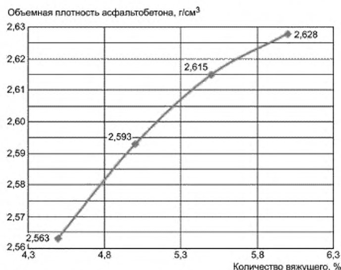
Рисунок Б.2 — Значение объемной плотности в зависимости от разного количества вяжущего
