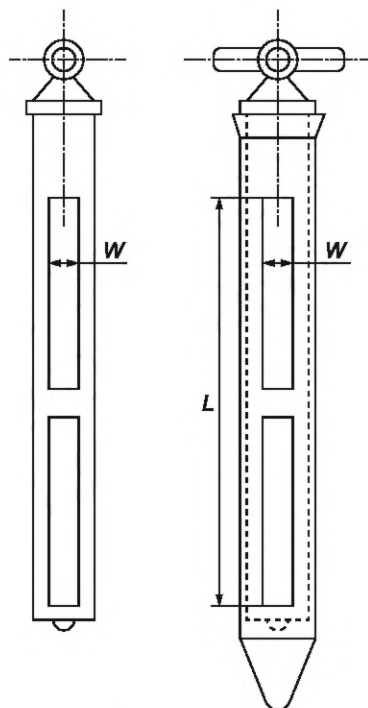
Рисунок 1 — Схема пробоотборной трубки
