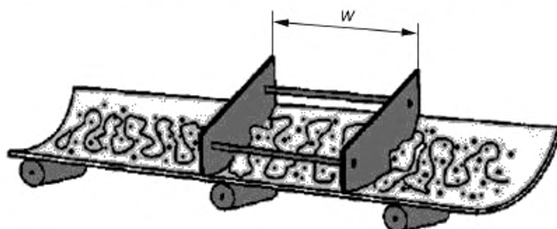
Рисунок 1 — Схема пробоотборной рамки
