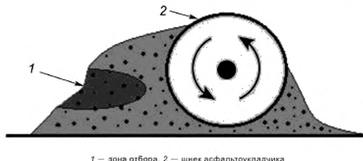
1 — зона отбора. 2 — шнек асфальтоукладчика
