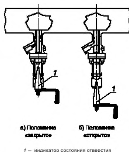
Рисунок 2 — Схема пробоборного крана поршневого типа
