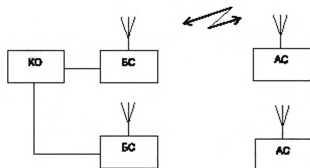
Рисунок 4.2 — Структурная схема организации многозонавой сети подвижной радиосвязи
