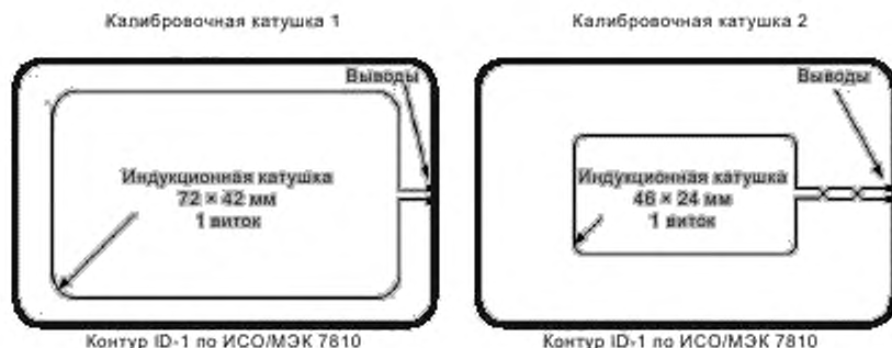
Рисунок 1 — Калибровочные катушки 1 и 2
