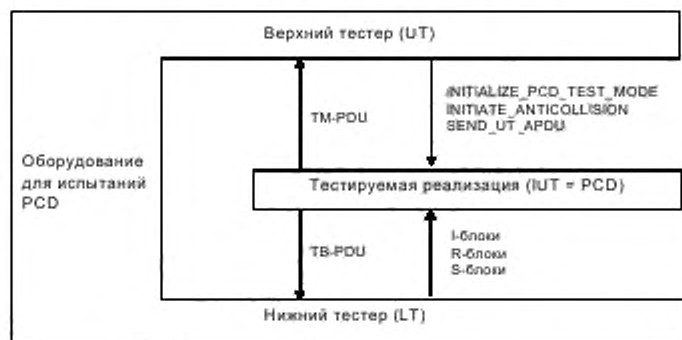
Рисунок Н.1 — Принципиальная архитектура тестера
