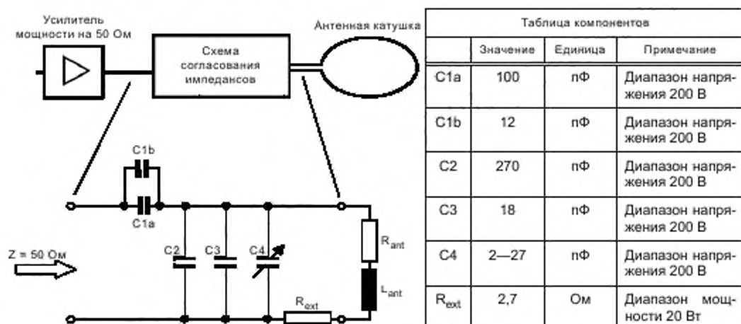
Рисунок A.9 — Схема согласования импедансов 2
