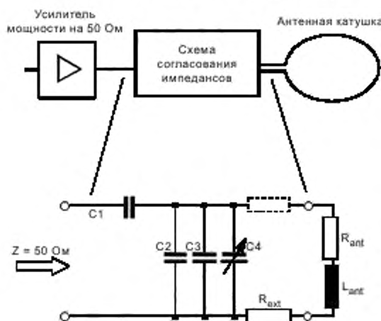
Рисунок А.5 — Схема согласования импедансов для скорости передачи fc/128
