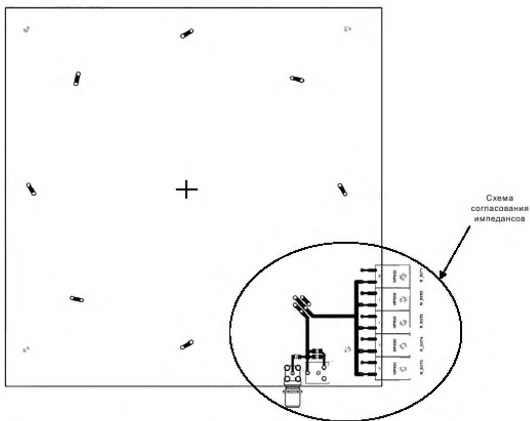
Рисунок A.1 — Топология испытательной антенны PCD 1, включающая в себя схему согласования импедансов для скорости передачи fc/128 (вид спереди)
